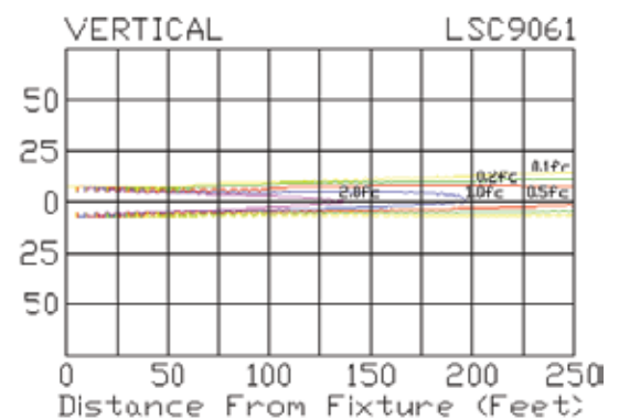
Par 36, 12V 30W Sealed Beam
