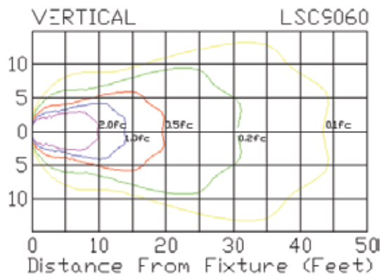
Par 36, 12V 25W Sealed Beam
