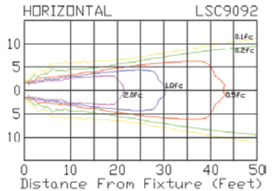
Par 36, 12V 12W Sealed Beam Halogen
